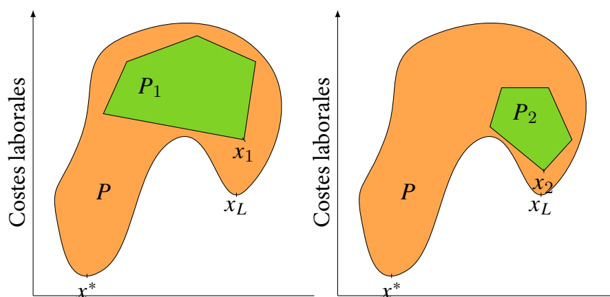
Figura 9: Gráficas representando los dos primeros pasos iterativos del método.
