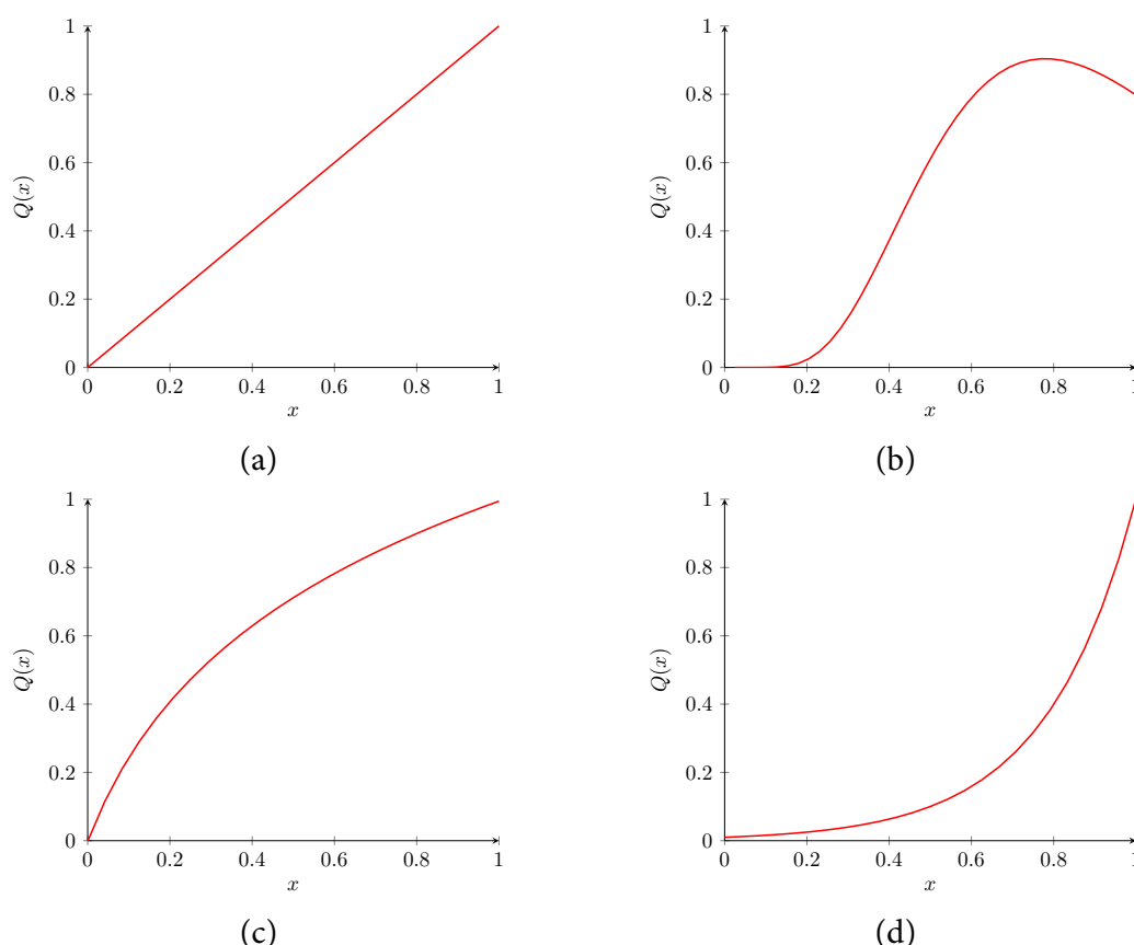
Figura 7: Ejemplos de funciones lineales (a), y no lineales (b,c,d). Si las entendemos como funciones de producción, el eje horizontal es la cantidad de insumos y el vertical la de productos.
