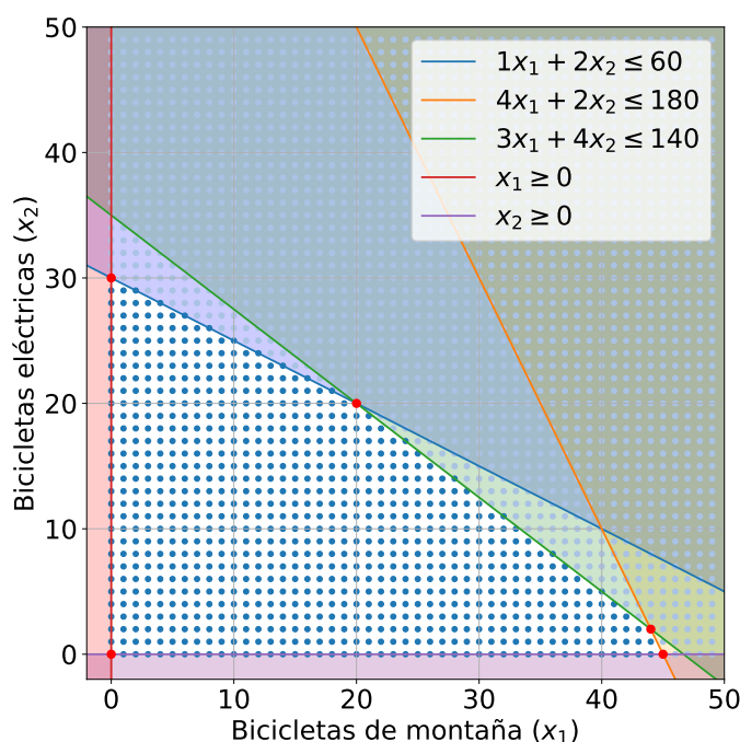
Figura 10: La zona en blanco representa la región factible del problema de programación lineal que aparecía de la Sección 3.2, mientras que los puntos en azul representan la región factible de su correspondiente versión entera, es decir, el problema de las bicicletas imponiendo la condición de que las variables sean números enteros (problema de programación lineal entera).
