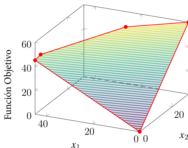
Figura 6: Valores de la función objetivo en la región factible, representada por el área delimitada por las líneas rojas. Nótese que la función tiene un valor constante en las rectas sombreadas en el interior del polígono (valor más bajo de color lila, más alto amarillo).
