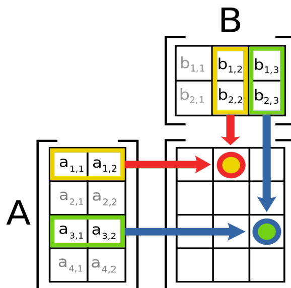
Figura 2: Ilustración gráfica del producto de matrices.
