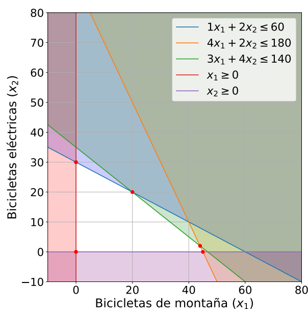
Figura 3: La región factible del problema de optimización es un poliedro. Los planos de diferentes colores corresponden a las restricciones del acero (azul), aluminio (naranja), horas de trabajo (verde) y no negatividad de la solución (rojo y violeta), respectivamente.
