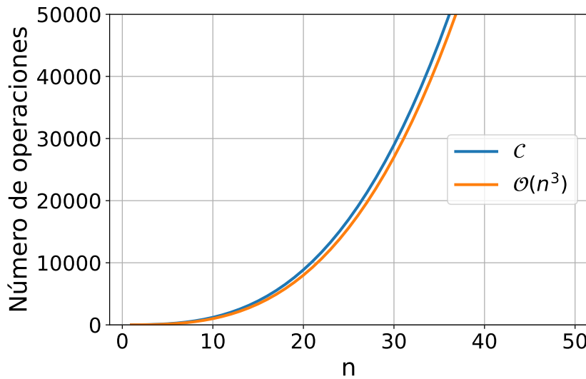
Figura 12: Comparación de la complejidad O(n^3) y número exacto de operaciones del método Gauss-Jordan.
