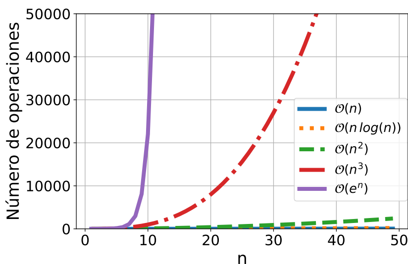
Figura 11: Evolución de la complejidad computacional en función de n .
