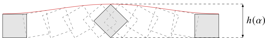
Figura 5: Ejemplo visual de los posibles máximos de un poliedro convexo sencillo (cuadrado) donde h(\alpha) es la altura en función del ángulo de inclinación. Los puntos más altos o son un vértice o una arista.
