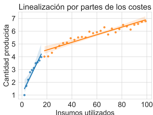
Figura 8: Ejemplo de costes marginales decrecientes. Aproximamos la nube de puntos por dos rectas, según se produzca más o menos cantidad. La zona sombreada nos indica el intervalo de confianza de la aproximación.
