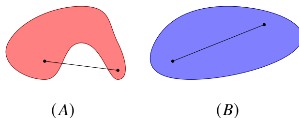
Figura 4: Ejemplo visual de un conjunto no convexo (A) y otro convexo (B).
